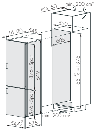
Einbaukühlschrank SMS-Norm / 55 cm 13/6 Classic
