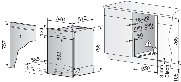
Geschirrspüler GS 55 Swiss Premium Line, SMS-Norm / Nischenbreite 55 cm
