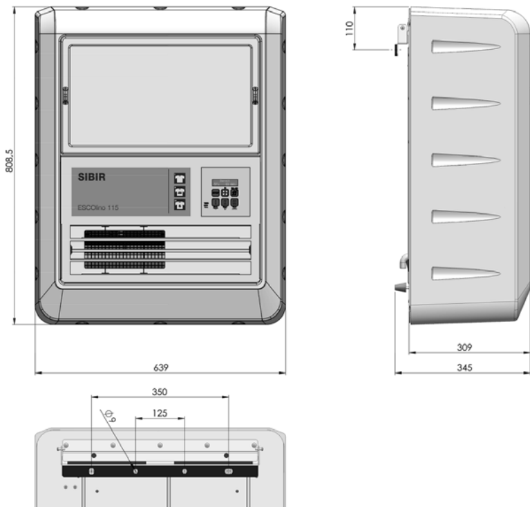
Abb. 2: Maßzeichnung
